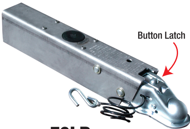
70LP Actuator
